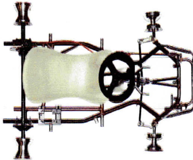
Вид сверху шасси в комплекте с рулевым управлением, педалями, топливным баком, полком, задней осью, колесными дисками, креплением двигателя (опционно), но без сиденья, шин, бамперов и кузова (Пластика) Insert plan view of chassis with complete steering, pedals, fuel tank, floor, rear axle, rims, engine support, but without seat, tyres, bumpers or bodywork
